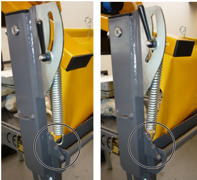
Pendelschneidarm-Feder, je nach Federspannung, in den 1., 2. oder 3. Haken einhängen Bild 4.14
