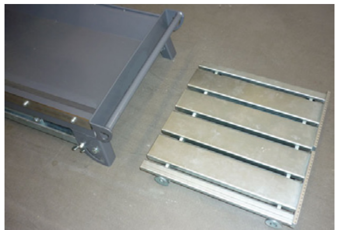
Rolltisch von der CTS•56 entfernt
