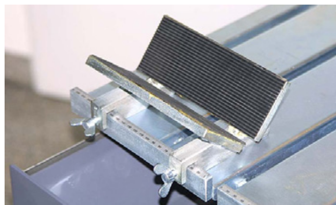
Prisma (auf Rolltisch-Anschlag geklemmt)
