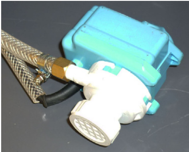
Wasserpumpe montiert
