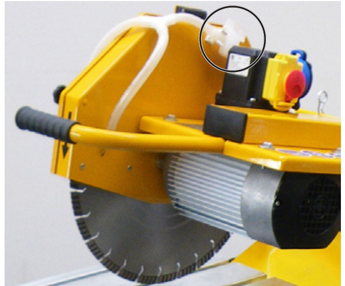
Beidseitiger Wasserzulauf im Trennscheibenschutz, stufenlos mit Absperrhahn regulierbar
