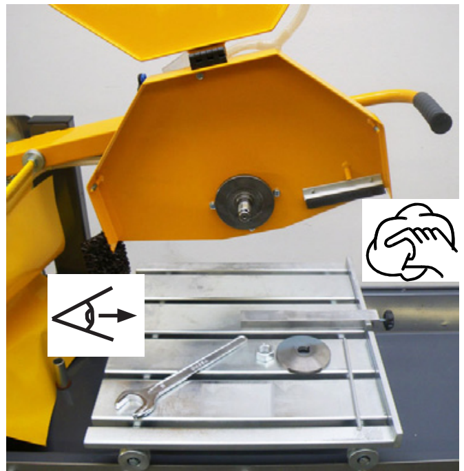
Schneidwellen-Mutter und Trennscheiben-Druckflansch demontiert
