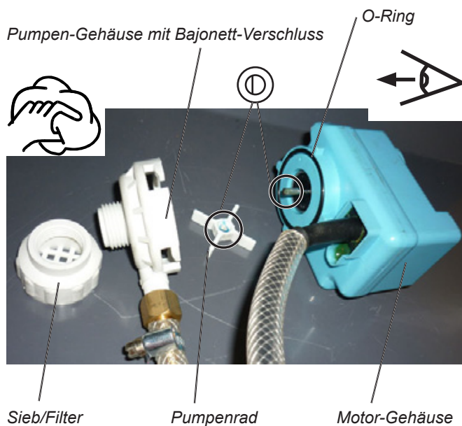
Wasserpumpe demontiert
