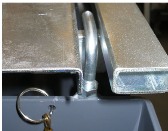
Rolltisch-Transportsicherung an Rolltisch ausgerichtet Bild 5.9
