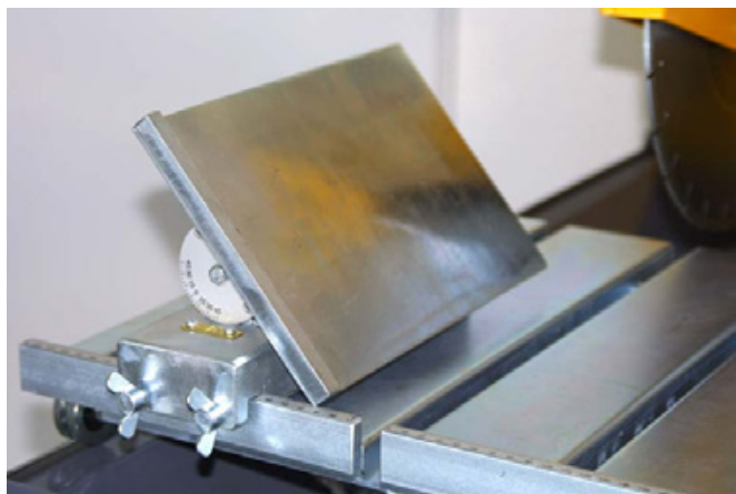
Jollytisch (auf Rolltisch-Anschlag geklemmt)
