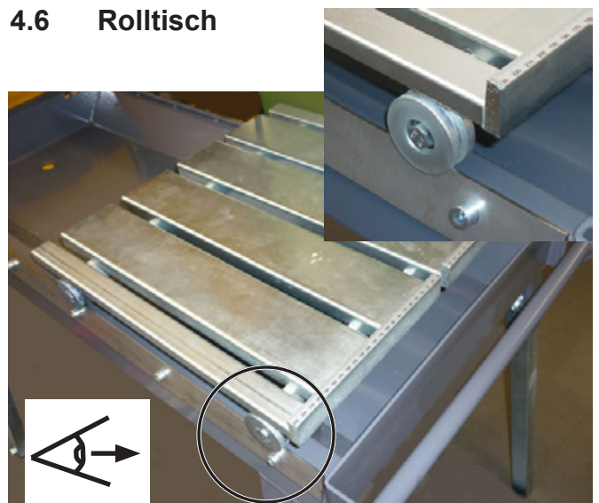
Rolltisch mit den Führungsrollen auf die Führungsschiene setzen
