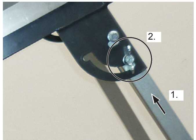
Standfuß einrasten, Flügelschraube festziehen
