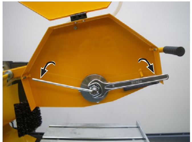
Schneidwellen- (Spann-) Mutter lösen
