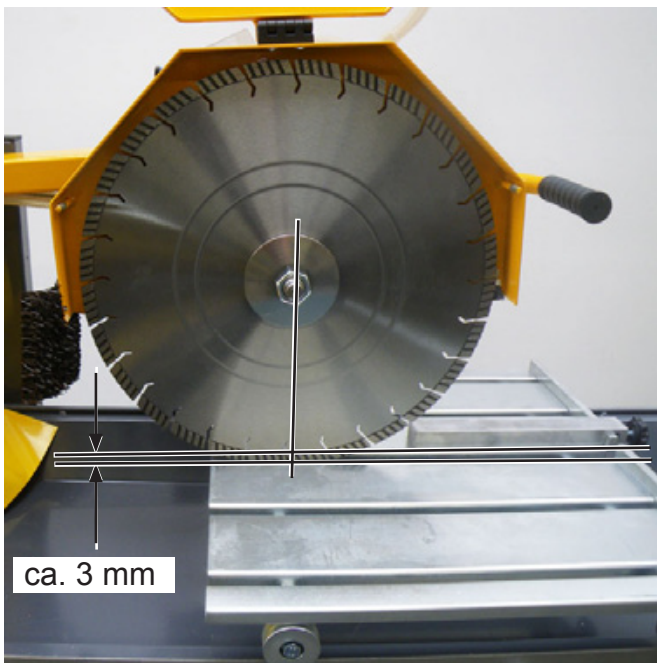
Pendelschneidarm (Trennscheibe) auf die maximale Schnitt-Tiefe eingestellt Bild 4.35
