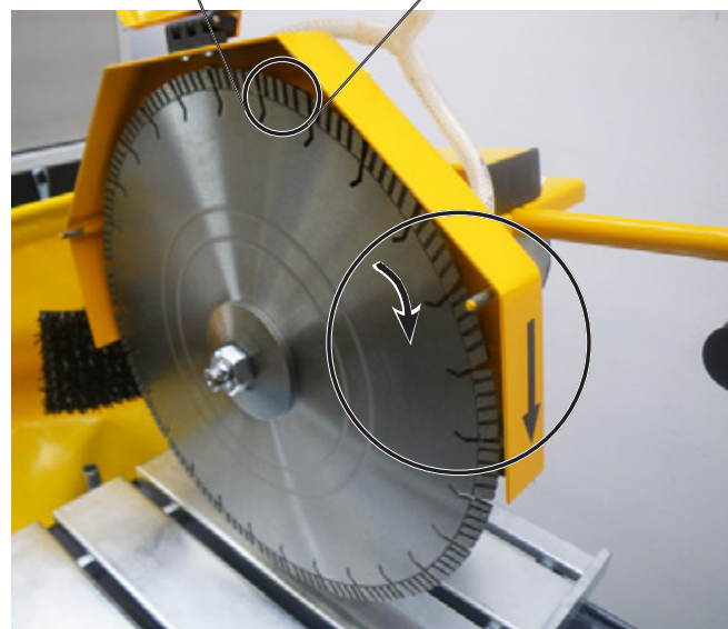
Diamant-Trennscheibe mit der Schneidrichtung der Diamant-Segmente entsprechend der Drehrichtung der Schneidwelle montieren Bild 4.31
