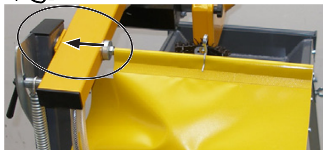
Spiel aus der Pendelschneidarm-Schwenkachse nehmen; Schwenk-Bolzen in Lagerung drücken Bild 5.6
