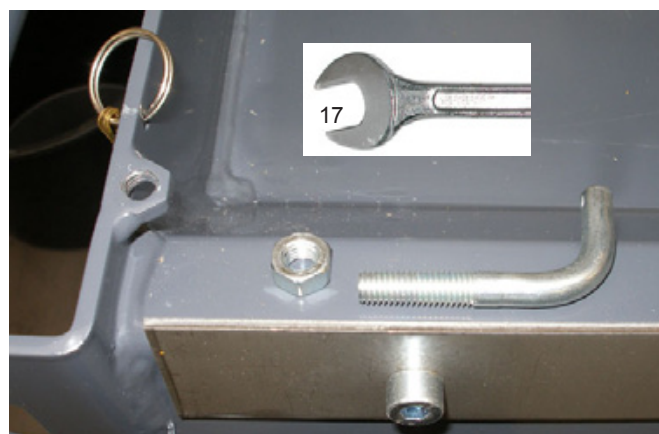
Rolltisch-Transportsicherung demontiert Bild 5.8
