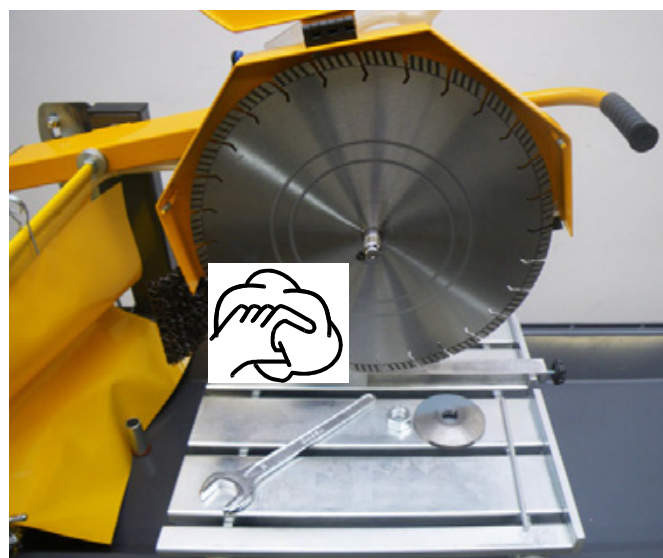
Diamant-Trennscheibe auf die Schneidwelle gesetzt Bild 4.29
