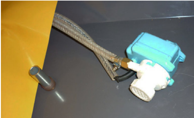
Überlaufstopfen im Abfluss der Wasserwanne, Wasserpumpe in der Wasserwanne
