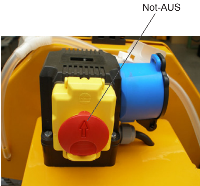
EIN/AUS, Not- AUS-Schalter, Klappe geschlossen Bild 4.40
