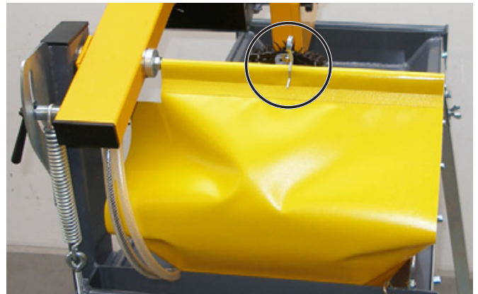
Spritzschutzplane montiert und mit dem Federstecker gesichert; Spritzschutzplane in die Wasserwanne stecken
