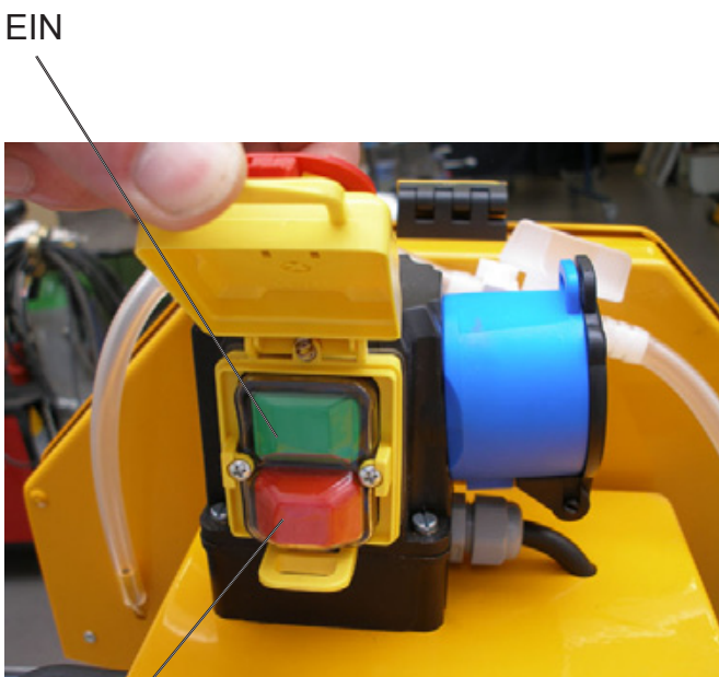
EIN/AUS, Not- AUS-Schalter, Klappe geöffnet Bild 4.41
