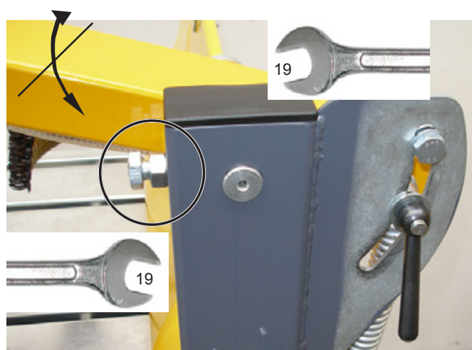
Spiel in der Pendelschneidarm-Schwenkachse; Sicherungsschraube mit Kontermutter am Schwenk-Bolzen Bild 5.5
