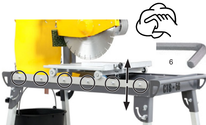
Rolltisch-Führungsleiste ausrichten
