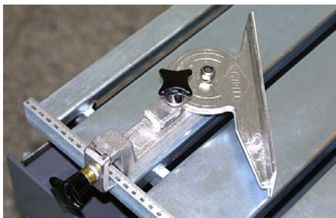
Winkelanschlag (auf Rolltisch-Anschlag geklemmt)
