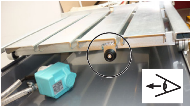
Rolltisch-Anstoßdämpfer, Wasserpumpe in Wasserwanne Bild 4.18
