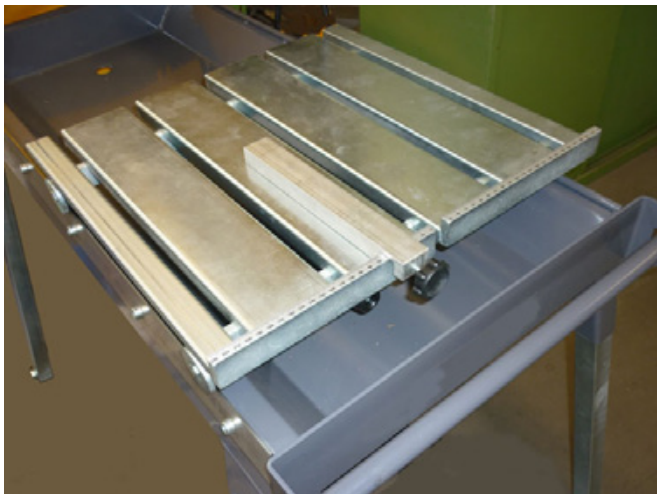
Seitenanschlag auf den Werkstückanschlag am Rolltisch klemmen Bild 4.19
